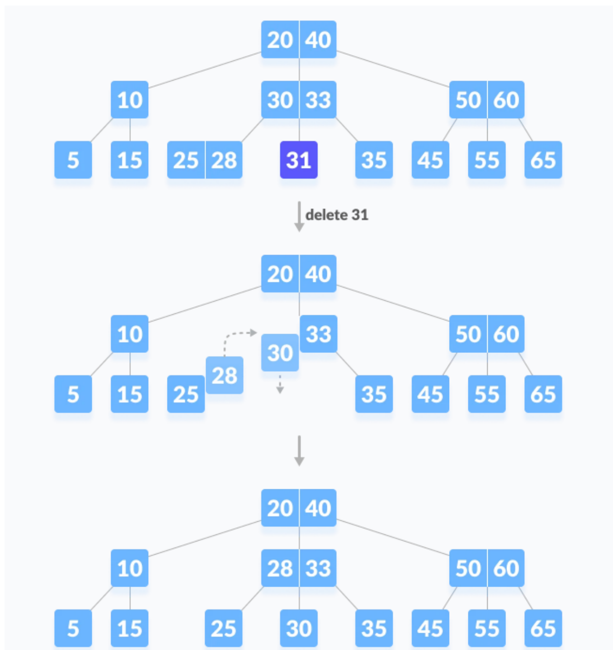
Figura 19: Árbol B
