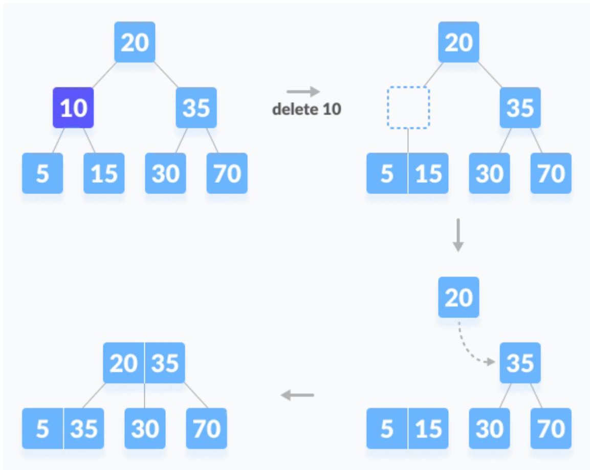
Figura 23: Árbol B
